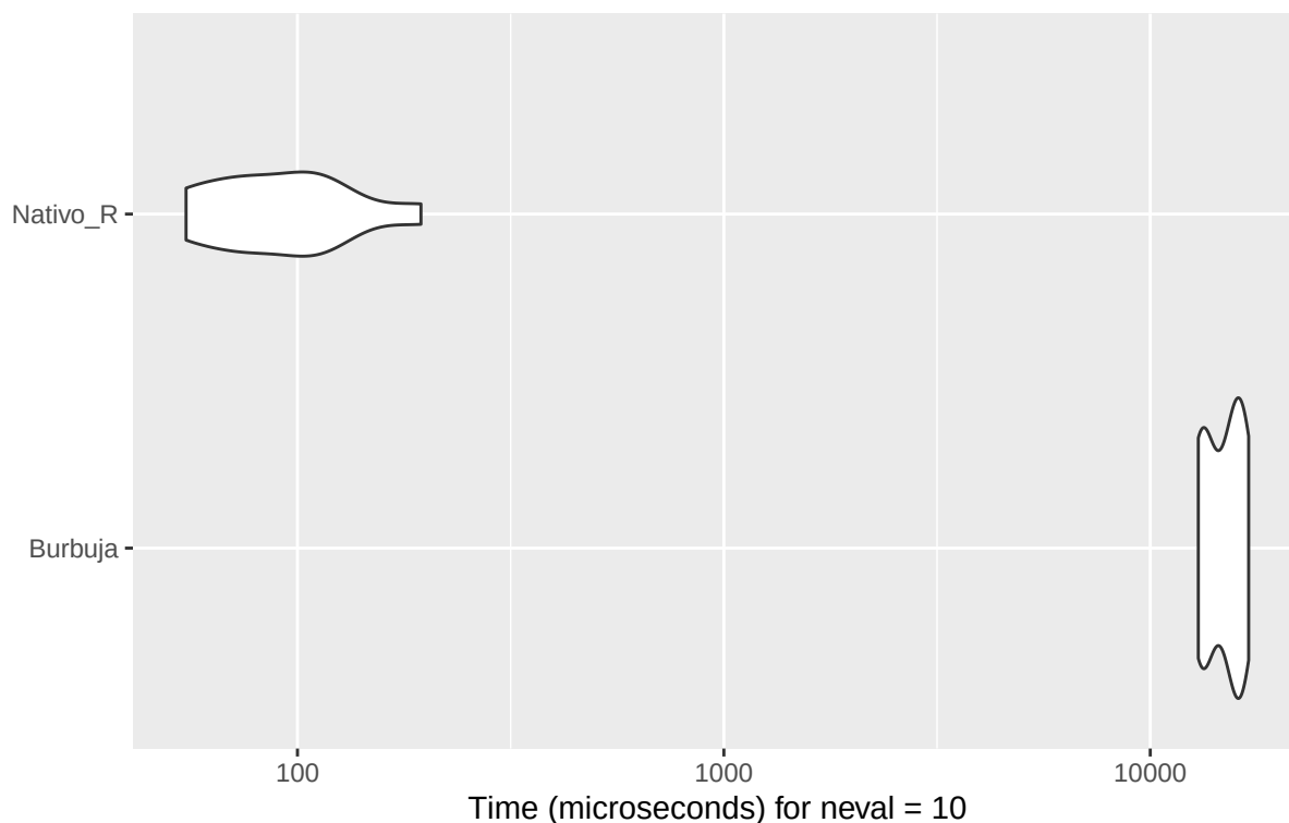
Distribución de tiempos: Burbuja vs Sort Nativo La escala suele ser logarítmica para apreciar la diferencia
